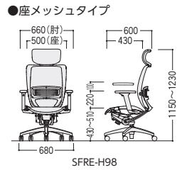
4軸シンクロロック機構 クラス最大の傾動範囲を実現したシンクロロック機構は、アルミ合金フレームにより背30°・座10°のダイナミックな動きを採用。ダイナミックな4軸メカとサスペンション・ファブリックが体を心地良くホールドします。また、ロックングストッパーによりベストポジションでの快適なパソコン作業をサポートします。
